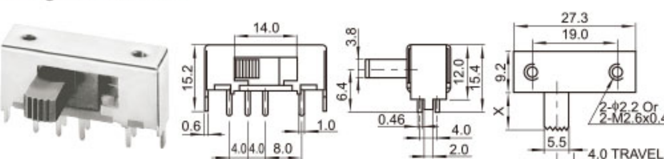
SK-23H01 (2P3T)
