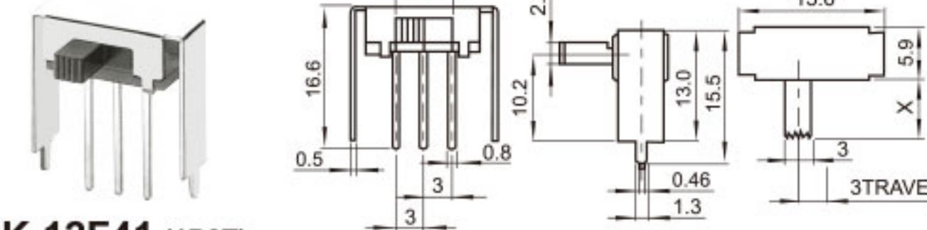
SK-12F41 (1P2T)
