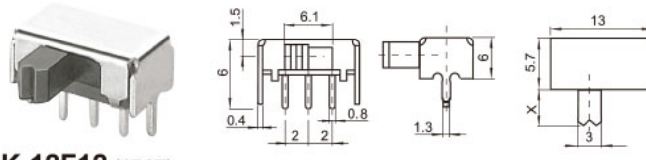
SK-12F12 (1P2T)
