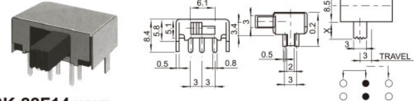
SK-22F14 (2P2T)
