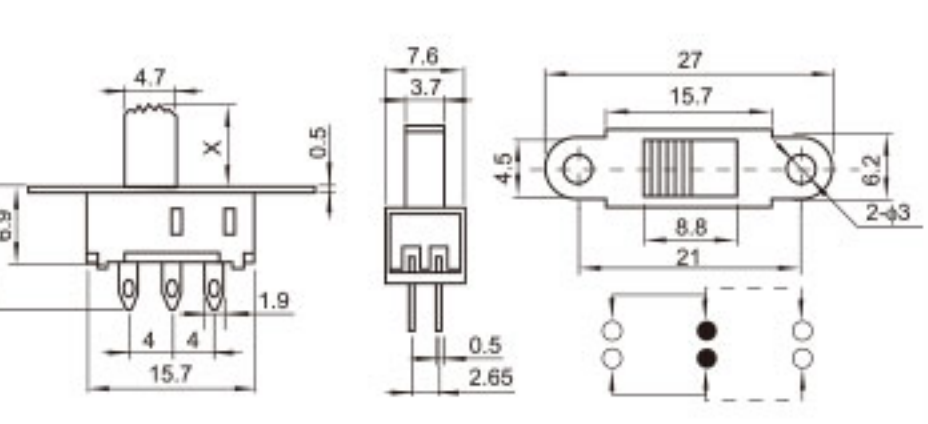
SS-22H03 (2P2T)
