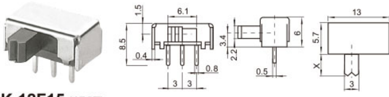
SK-12F15 (1P2T)
