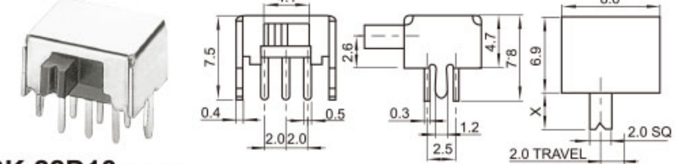
SK-22D13 (2P2T)
