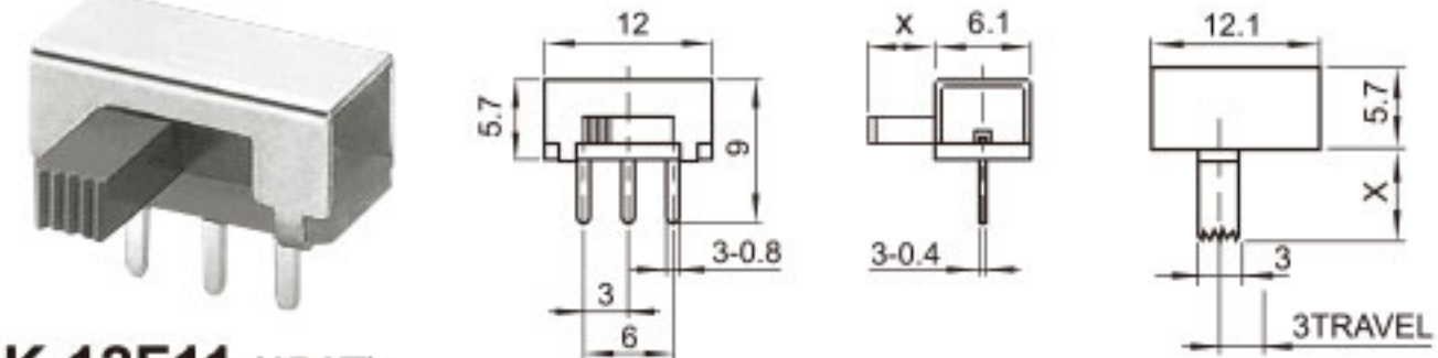
SK-12F11 (1P2T)
