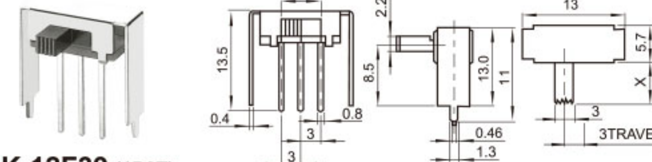
SK-12F39 (1P2T)
