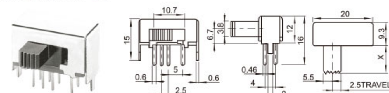
SK-23E01 (2P3T)
